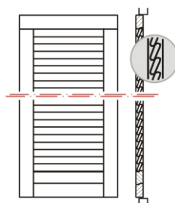
nepomična žaluzina sa zatvorenim leptirkama (nepomične leptirke)
